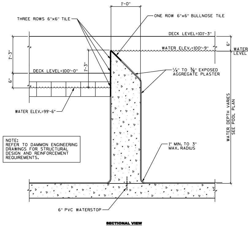
VANISHING EDGE WALL DETAIL 4 SCALE: 1" = 1'
