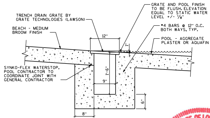
TRENCH SECTION A-A
