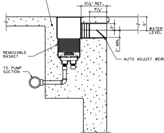
SKIMMER DETAIL 5 SCALE: 1" = 1'
