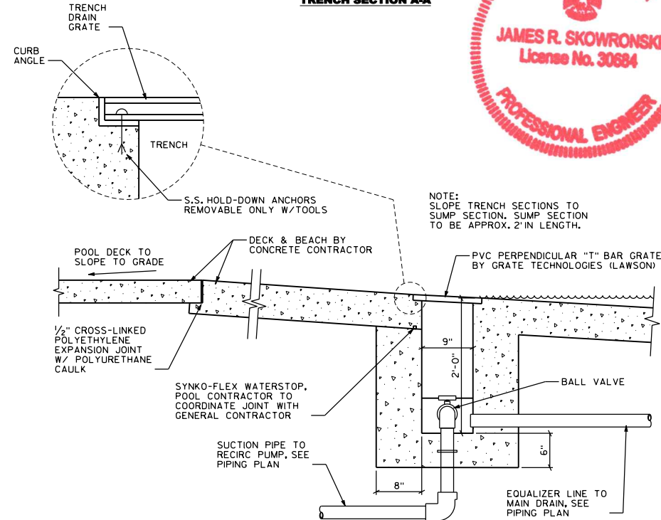
TRENCH SECTION A-A
