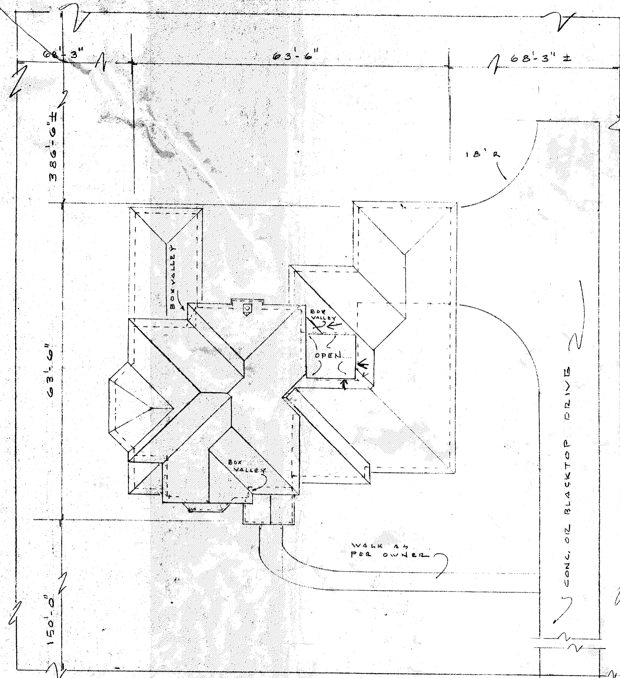
SITE PLAN 1"=10'
