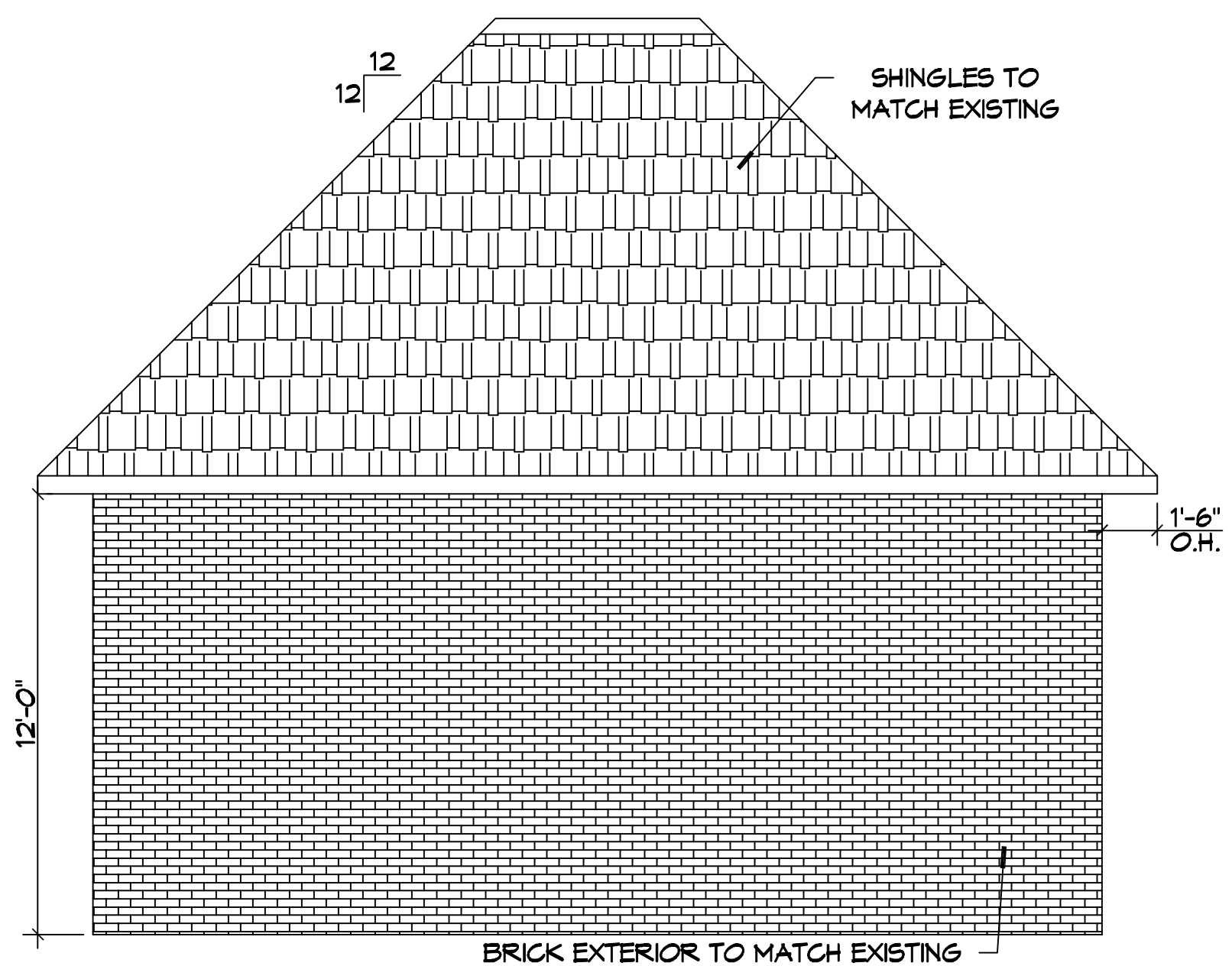
4 LEFT ELEVATION SCALE: 1/4"=1'-0"
