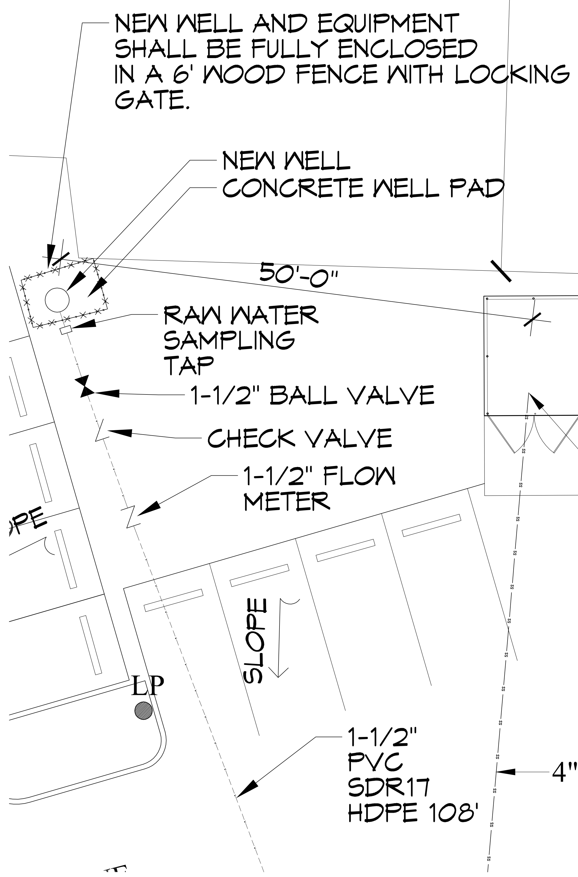
3 ENLARGED WELL PLAN SCALE: N.T.S.
