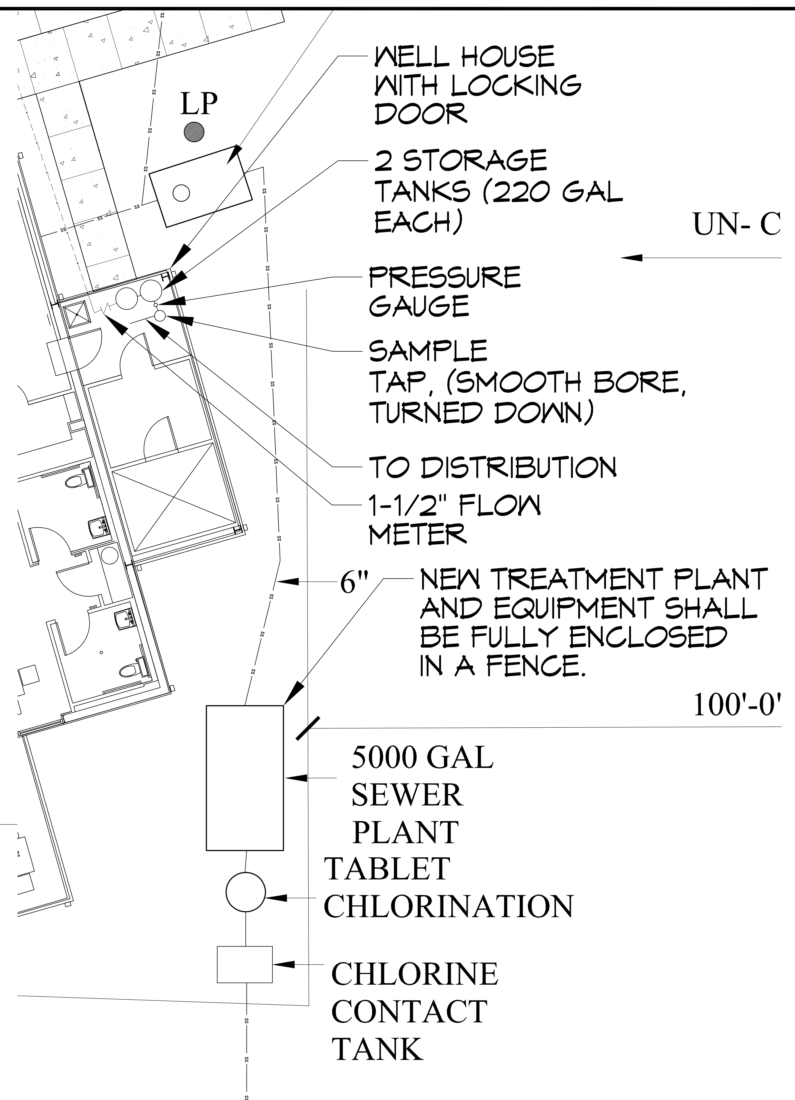
4 ENLARGED WELL PLAN SCALE: N.T.S.
