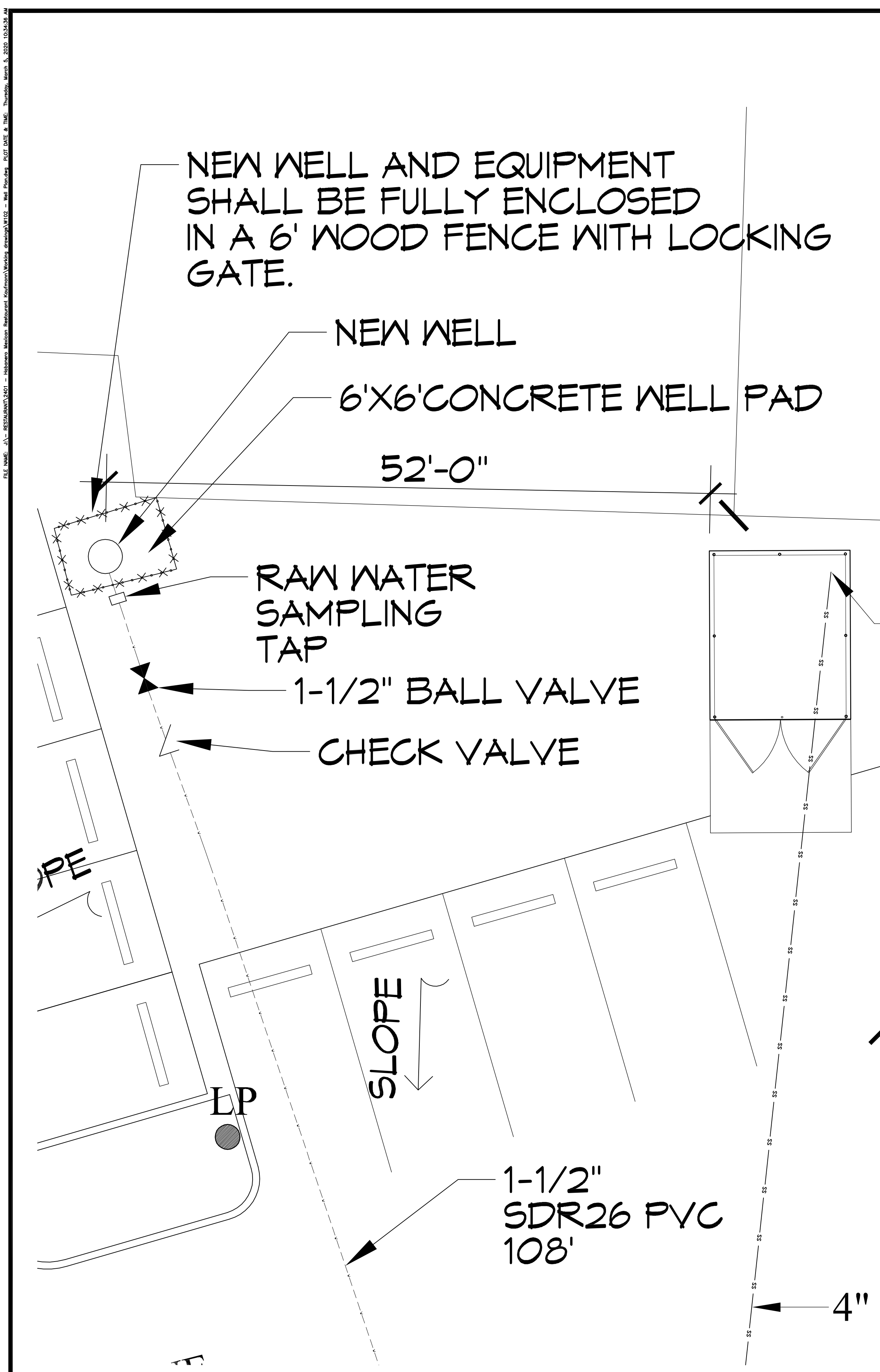
3 ENLARGED WELL PLAN SCALE: N.T.S.
