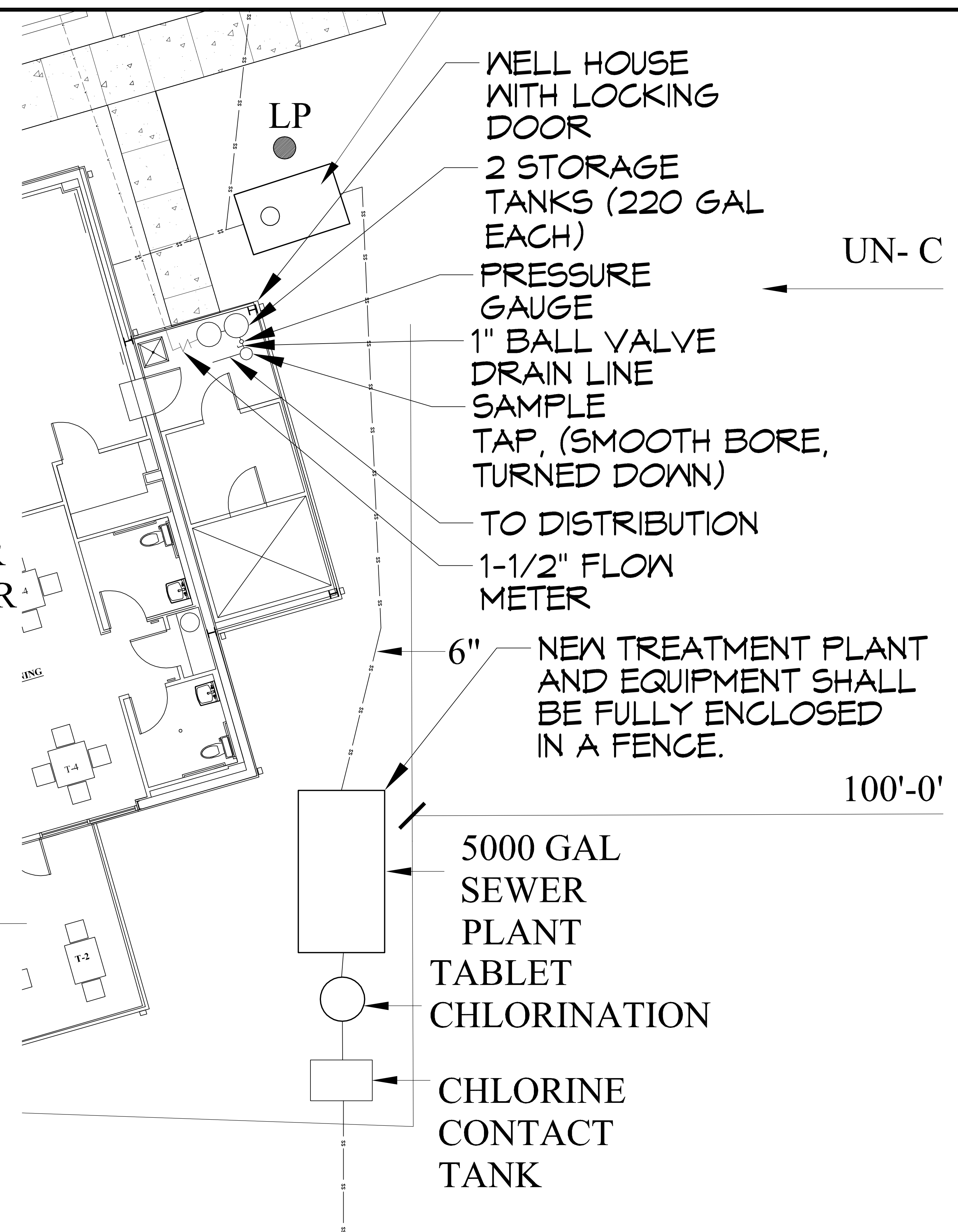
4 ENLARGED WELL PLAN SCALE: N.T.S.
