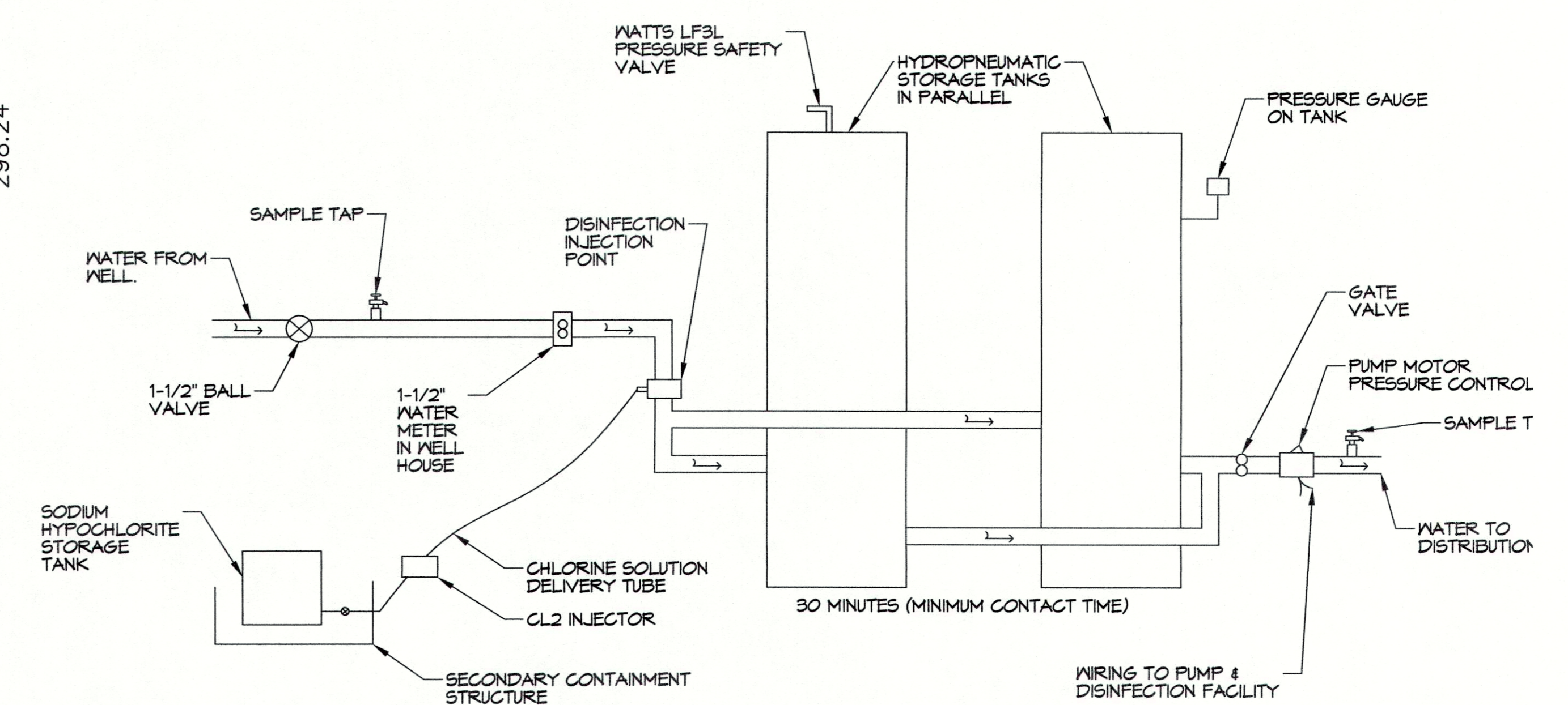
3 SMALL WATER SYSTEM CONFIGURATION SCALE: N.T.S.
