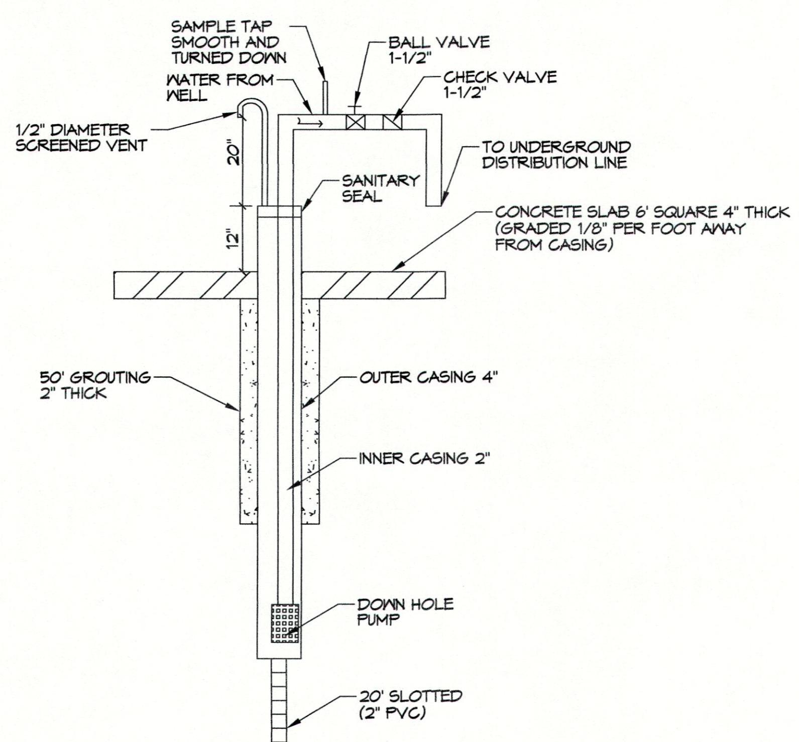
2 WELL HEAD SCALE: N.T.S.
