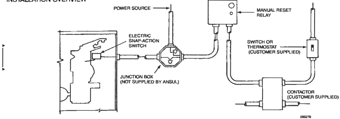
WIRING SCHEMATIC
