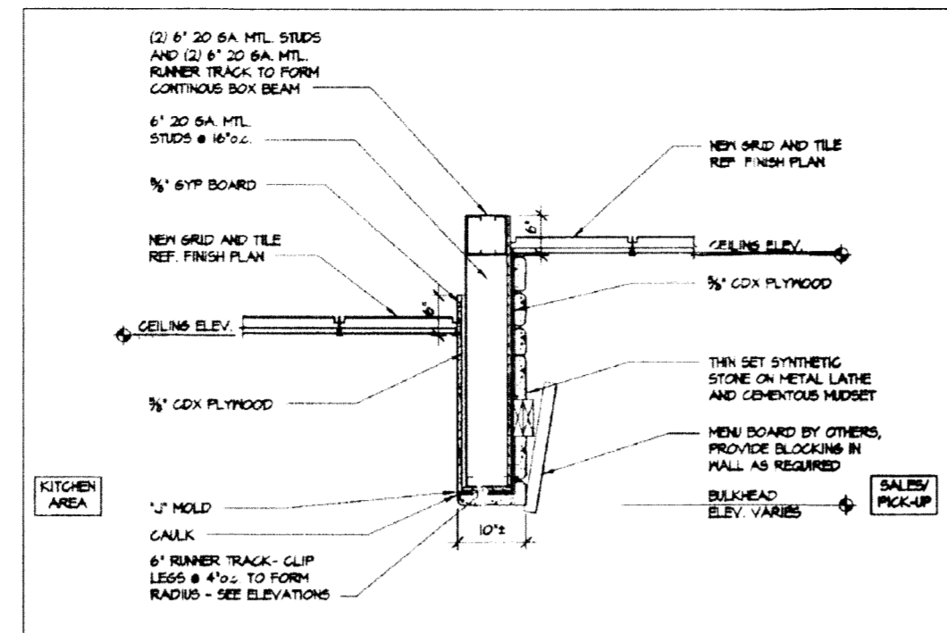
STONE ARCH SECTION SCALE: N.T.S.
