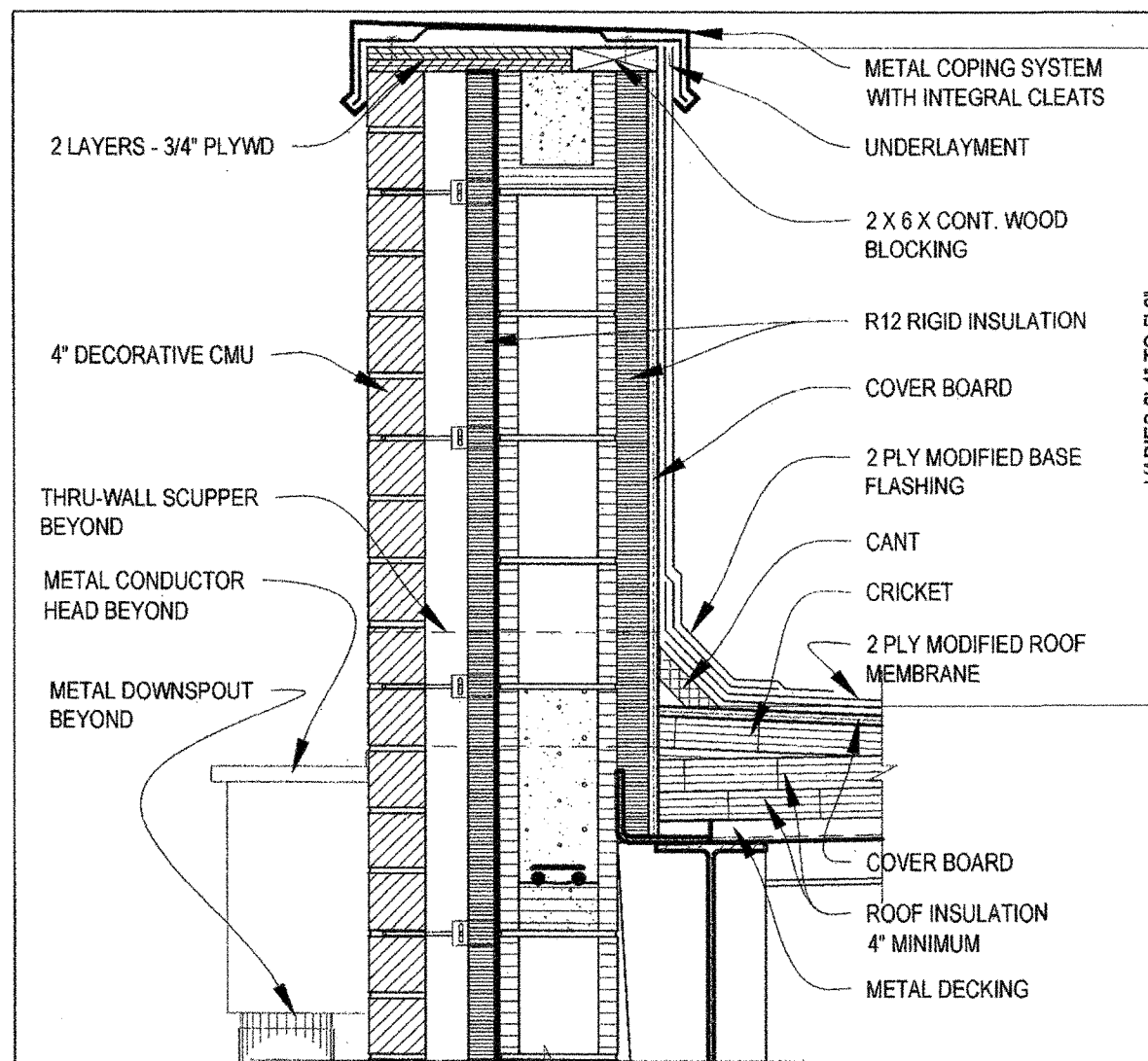
17 ROOF DETAIL A1.06 SCALE: 1" = 1'-0"
