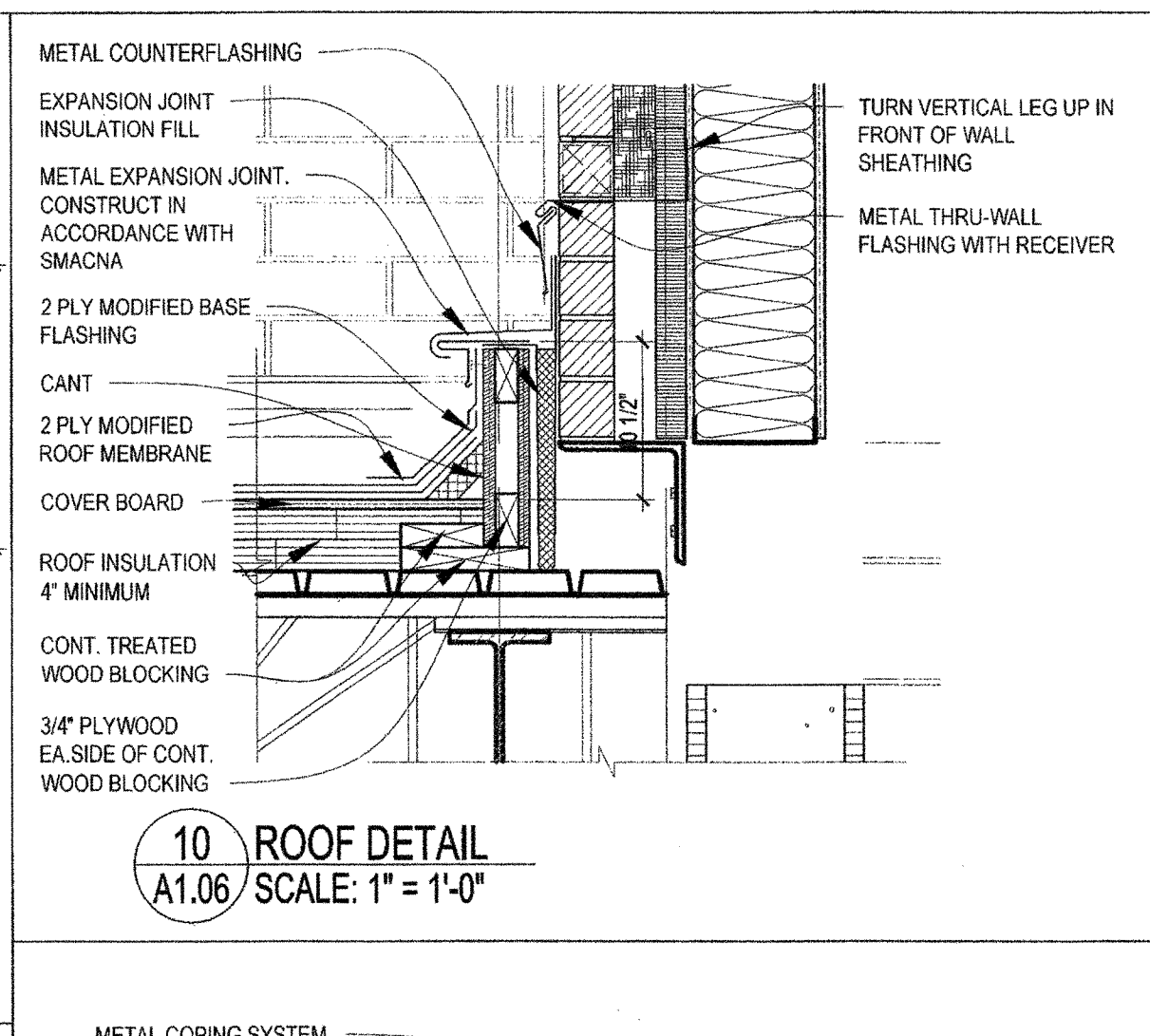
13 ROOF DETAIL A1.06 SCALE: 1" = 1'-0"
