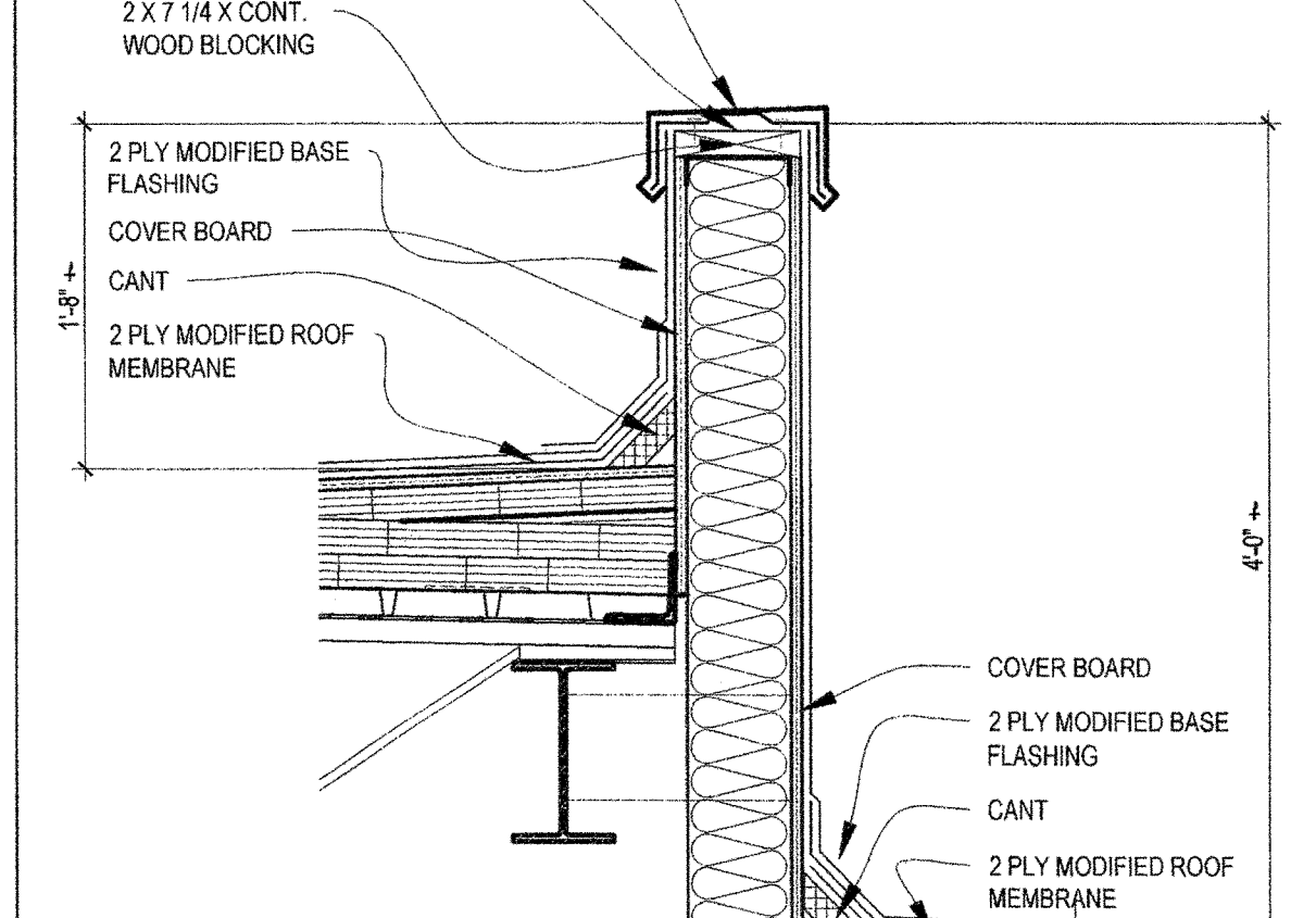
12A ROOF DETAIL A1.06 SCALE: 1" = 1'-0"
