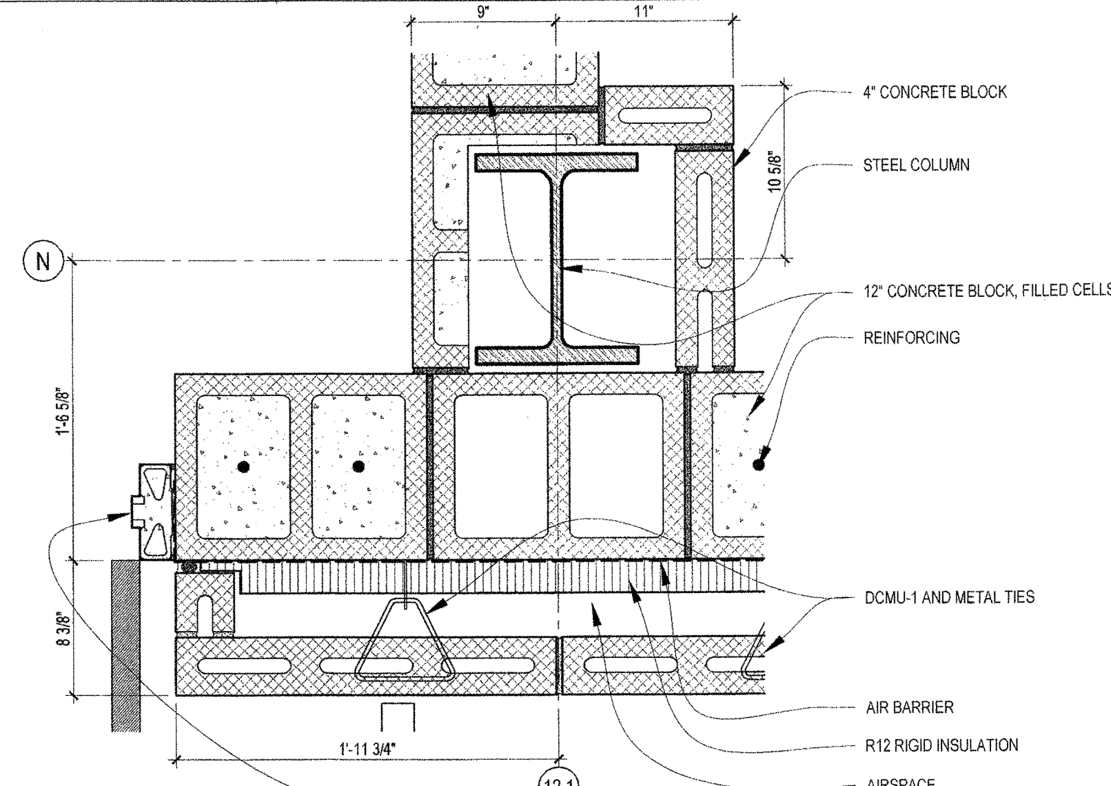
3 DETAIL A5.03 SCALE: 1 1/2" = 1'-0"
