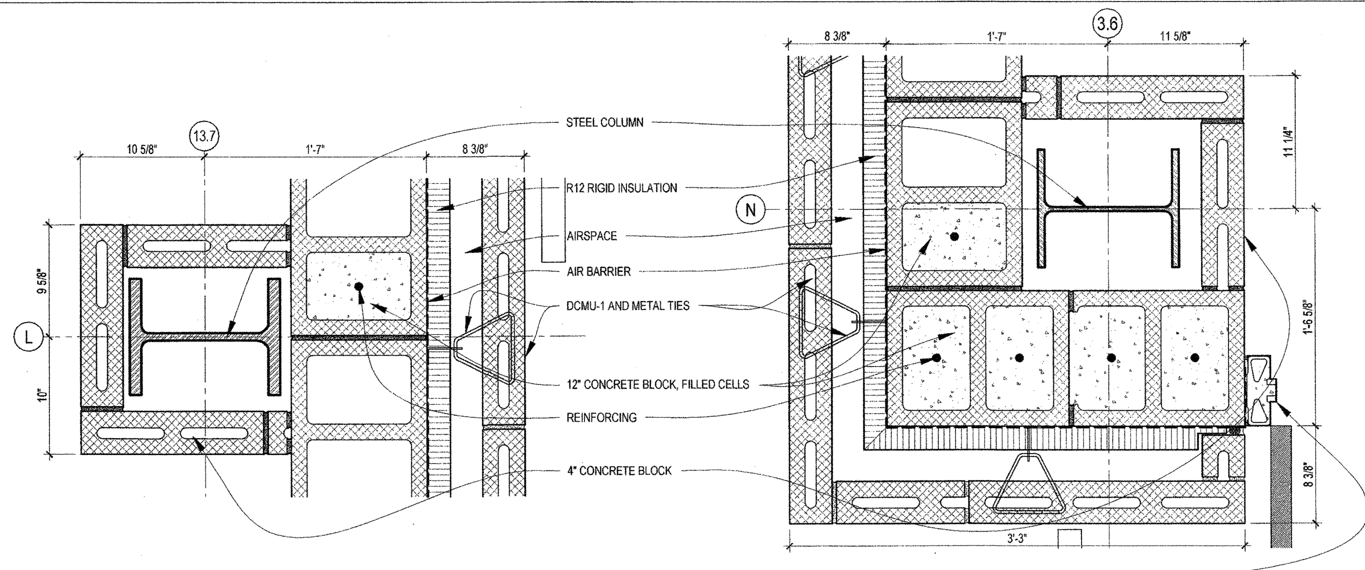
1 DETAIL A5.03 SCALE: 1 1/2" = 1'-0"
