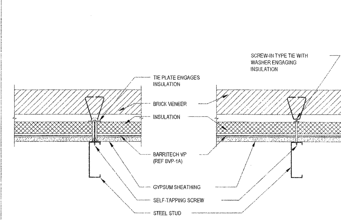
11 AIR BARRIER DETAIL - BRICK TIES III A5.11 SCALE: N.T.S
