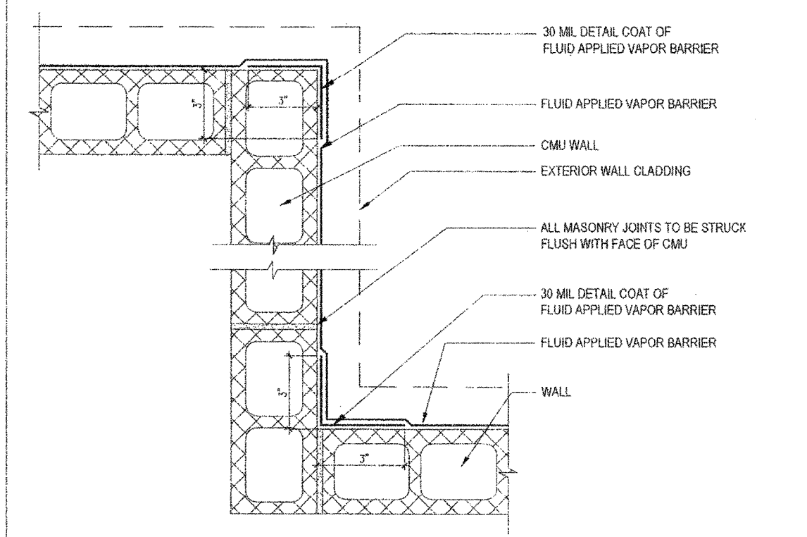
15 AIR BARRIER DETAIL - INSIDE/OUTSIDE CORNERS A5.11 SCALE: N.T.S
