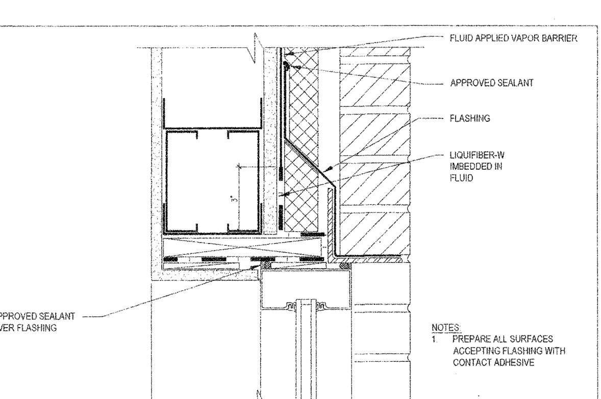
4 AIR BARRIER DETAIL - STOREFRONT - HEAD A5.11 SCALE: N.T.S
