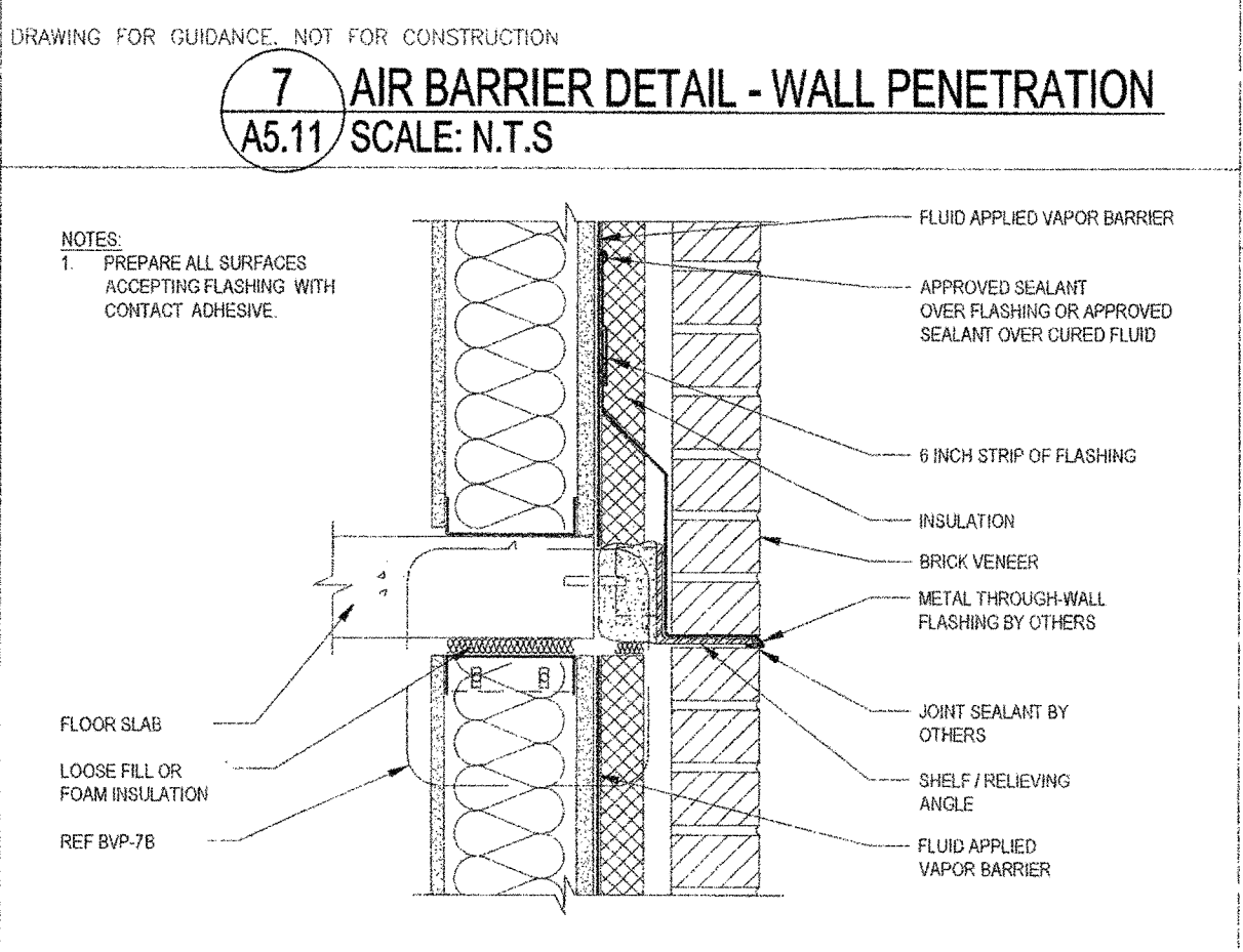
6 AIR BARRIER DETAIL - SHELF ANGLE A5.11 SCALE: N.T.S
