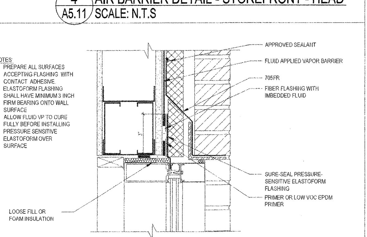
3 AIR BARRIER DETAIL - CURTAIN WALL - HEAD A5.11 SCALE: N.T.S
