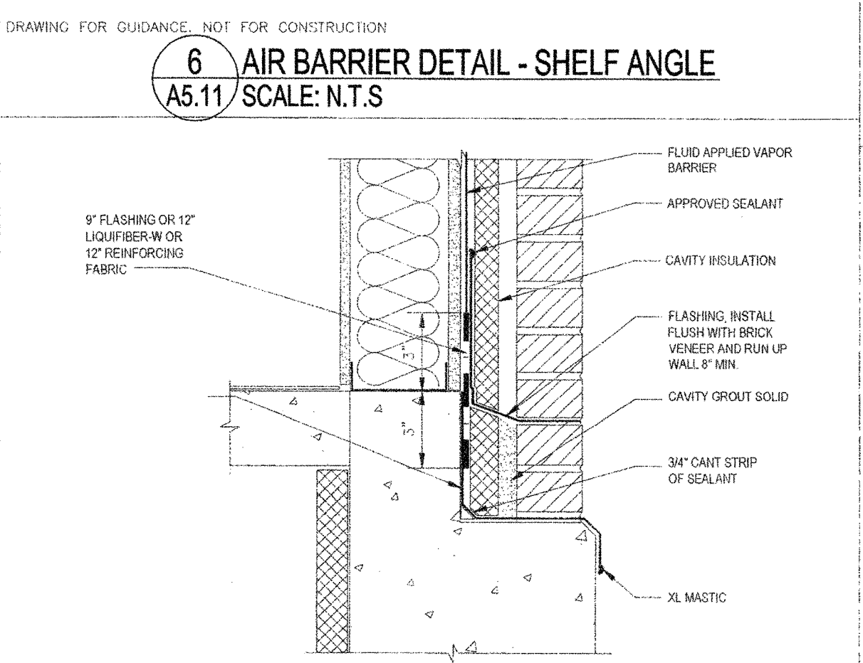
5 AIR BARRIER DETAIL - BRICK LEDGE A5.11 SCALE: N.T.S
