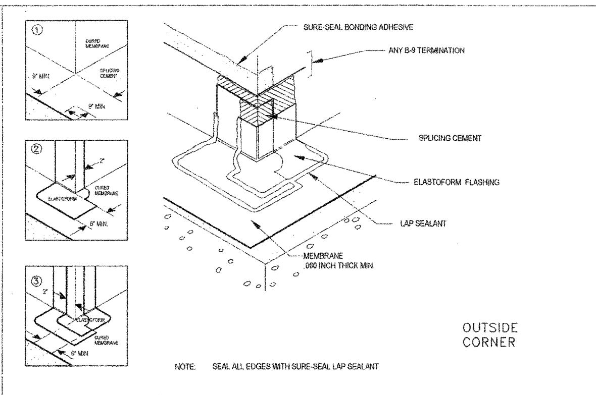
12 AIR BARRIER DETAIL - FIELD CORNER A5.11 SCALE: N.T.S
