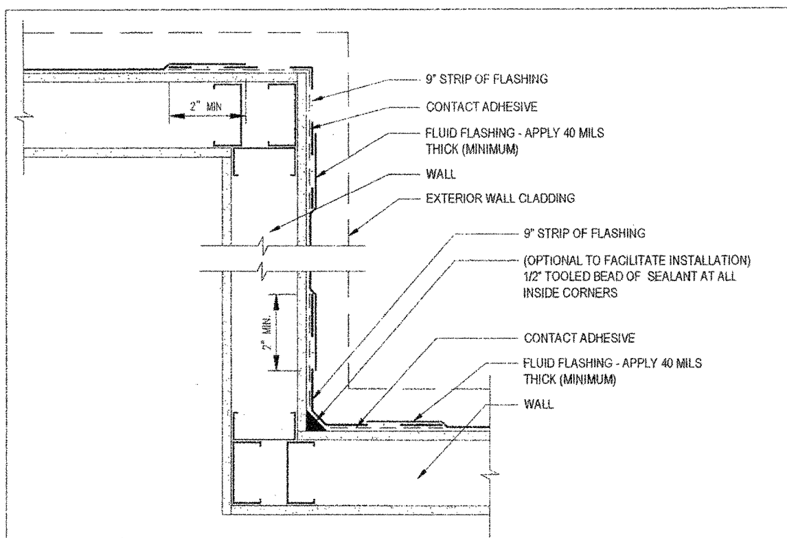
16 AIR BARRIER DETAIL - INSIDE/OUTSIDE CORNERS A5.11 SCALE: N.T.S
