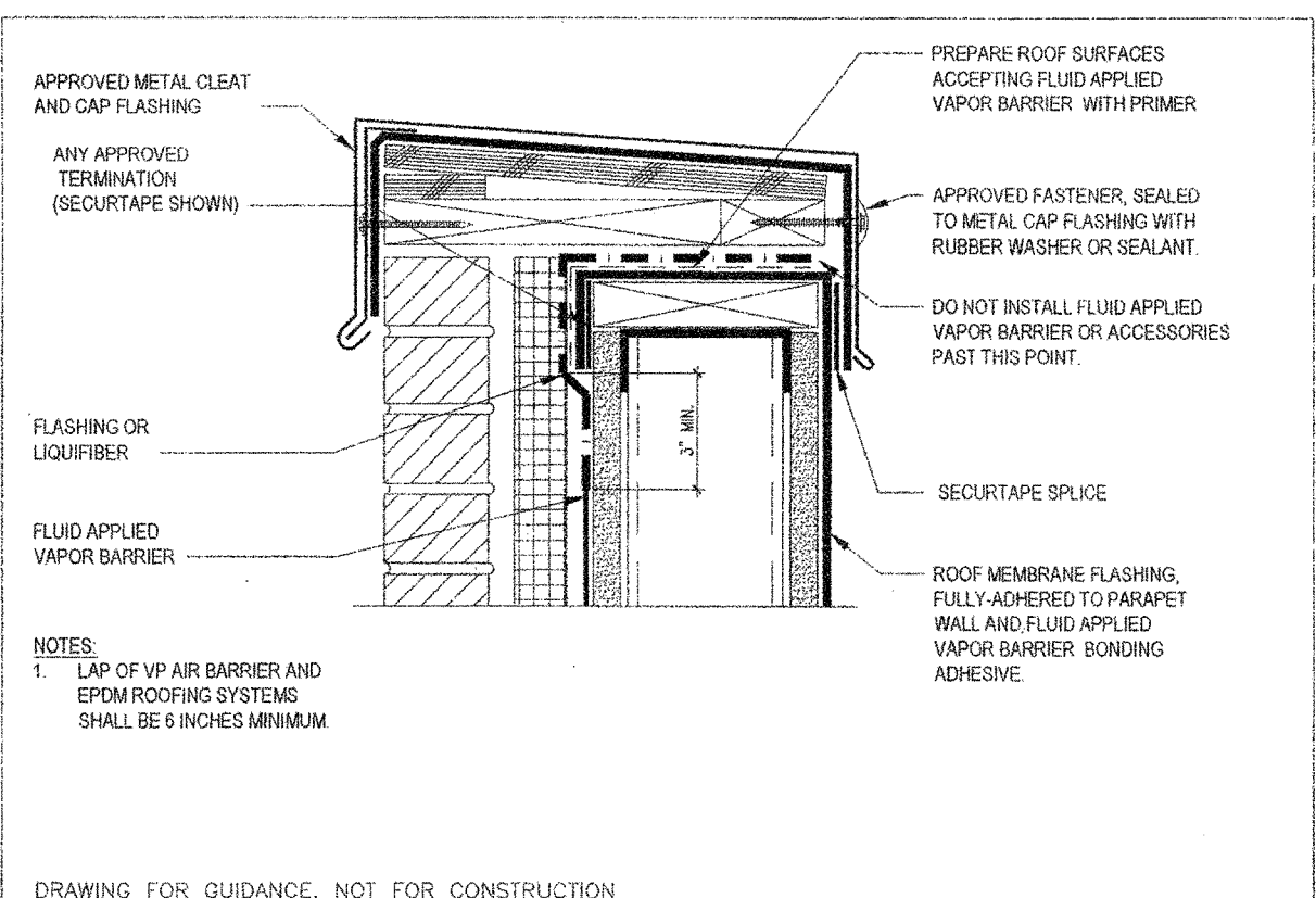
8 AIR BARRIER DETAIL - ROOF CAP TIE-IN A5.11 SCALE: N.T.S
