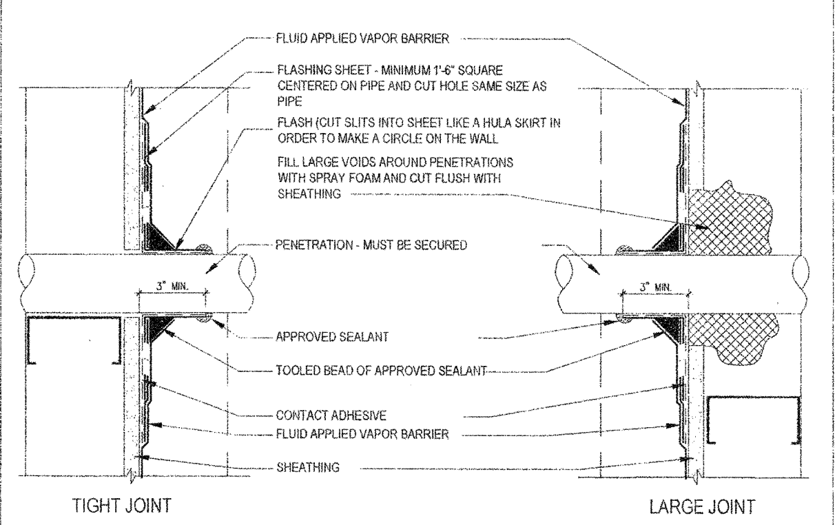
7 AIR BARRIER DETAIL - WALL PENETRATION A5.11 SCALE: N.T.S
