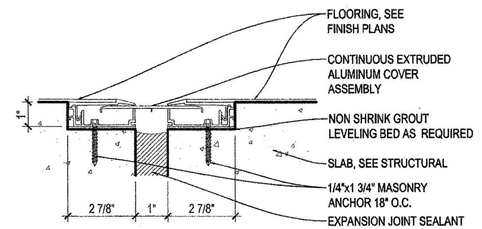
D E.J. FLOOR COVER A1.14 / SCALE: 3" = 1'-0"
