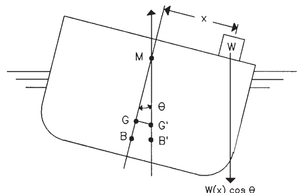
FIG. 2 Metacentric Height
