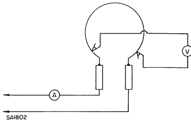
FIG. A1.1 Test Apparatus
