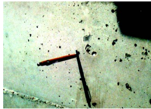
Fig. 2.3.3—Bugholes.
