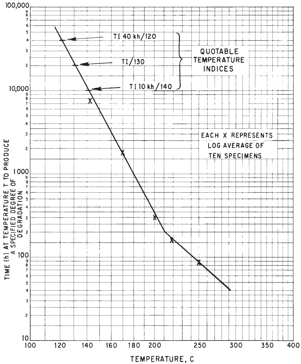
(SCALE : - 1/T ABSOLUTE) FIG. 6 Model Arrhenius Plot
