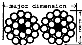
FIG. 1 Dimensions
