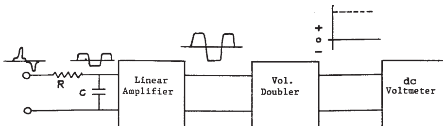
FIG. X1.1 R-C Integrator-Amplifier
