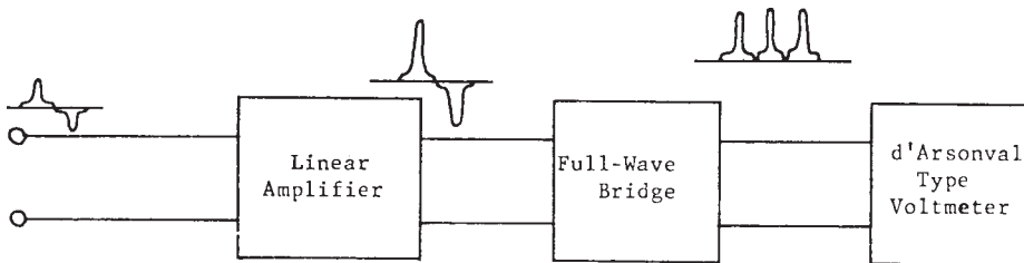
FIG. X1.3 Rectifier-Integrator
