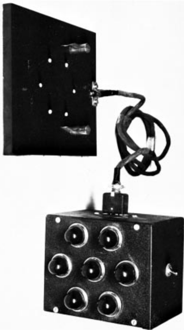
FIG. 4 Exudation-Indicator Device
