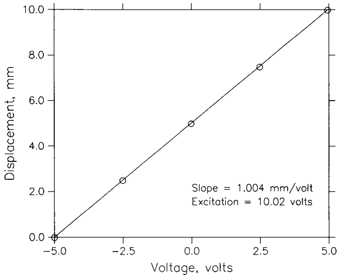
FIG. 2 LVDT Calibration
