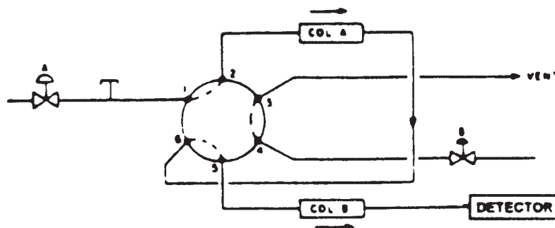
(b) Backflush
