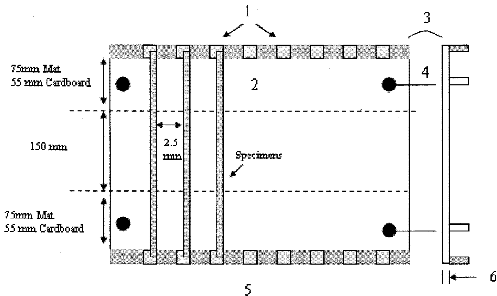
FIG. 4 St Tatbvic Brng Templakter Bar
