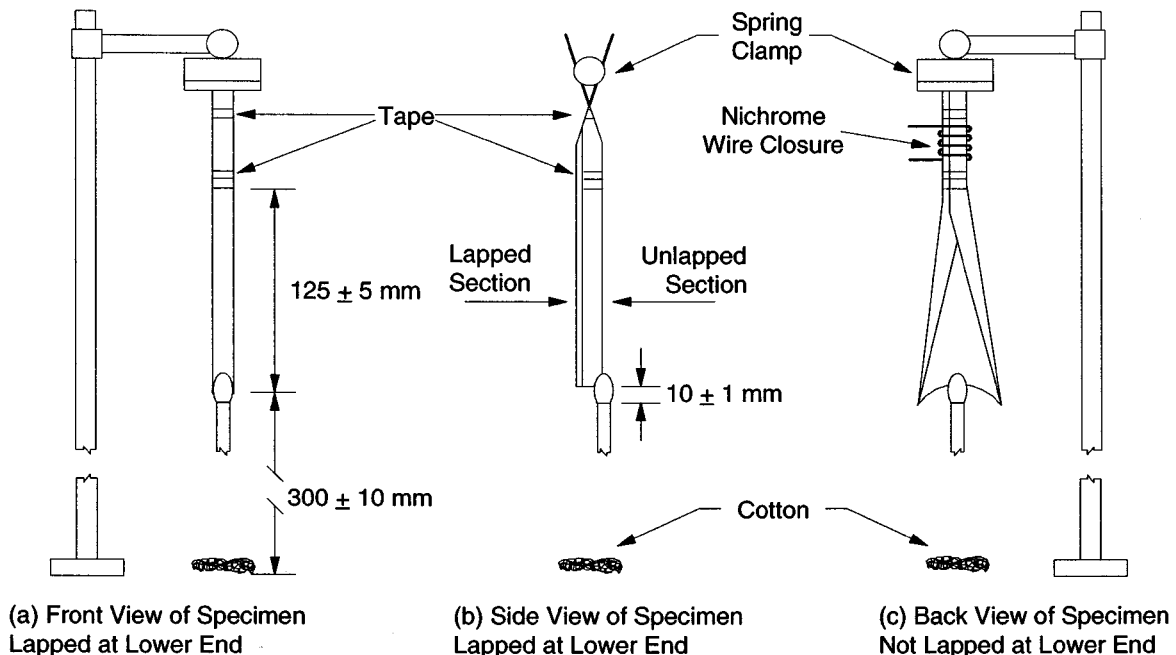
FIG. 1 Test Apparatus
