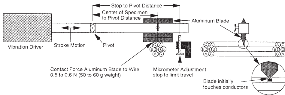
FIG. 25 Apparatus
