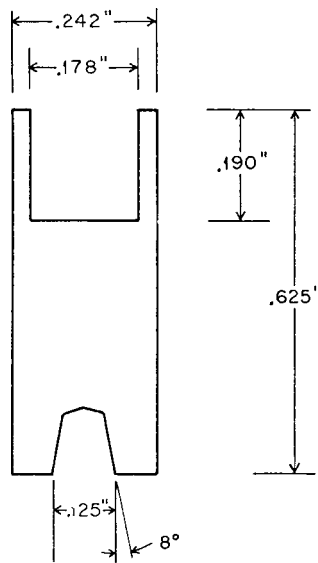
FIG. 3 Anode Cap 10
