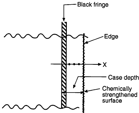
FIG. 2 Case Depth
