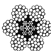
6 x 25 FILLER WIRE
