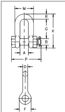
G-2150 / S-2150
