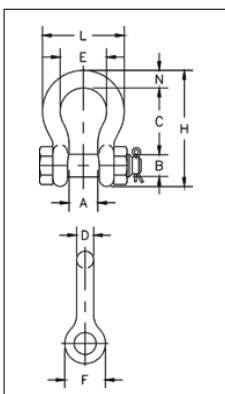
G-2130 / S-2130
