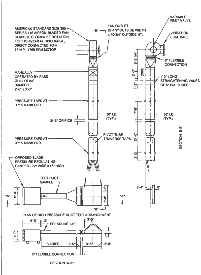
FIG. 7-4 TEST APPARATUS
