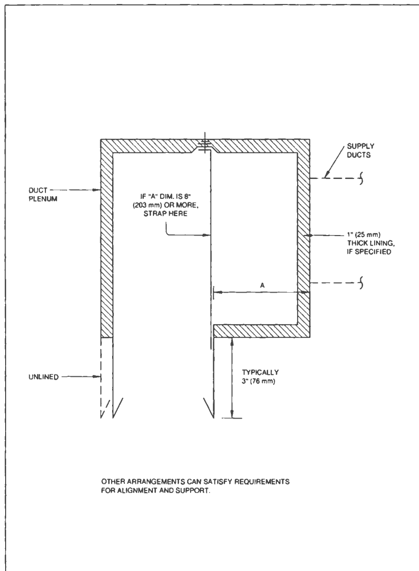
FIG. 2-16 LINEAR DIFFUSER PLENUM
