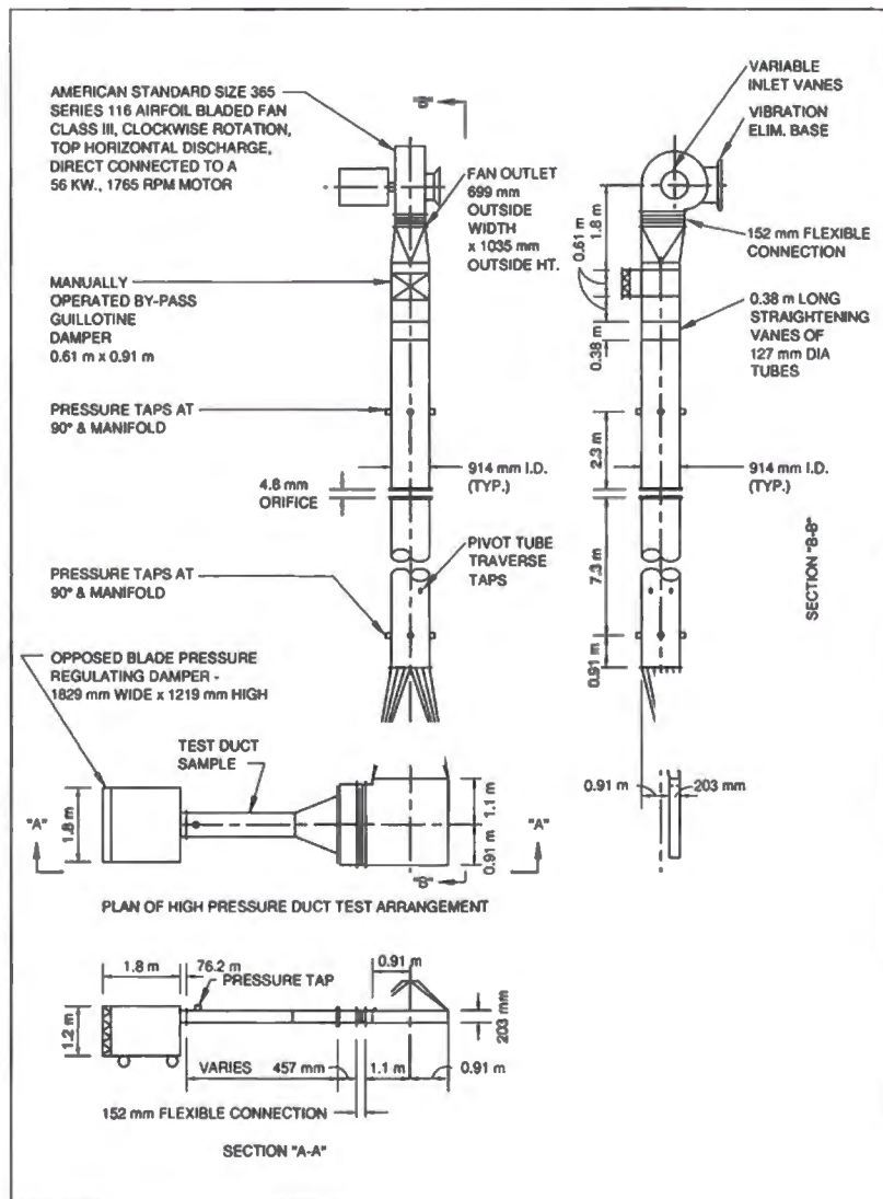
FIG. 7-4M TEST APPARATUS
