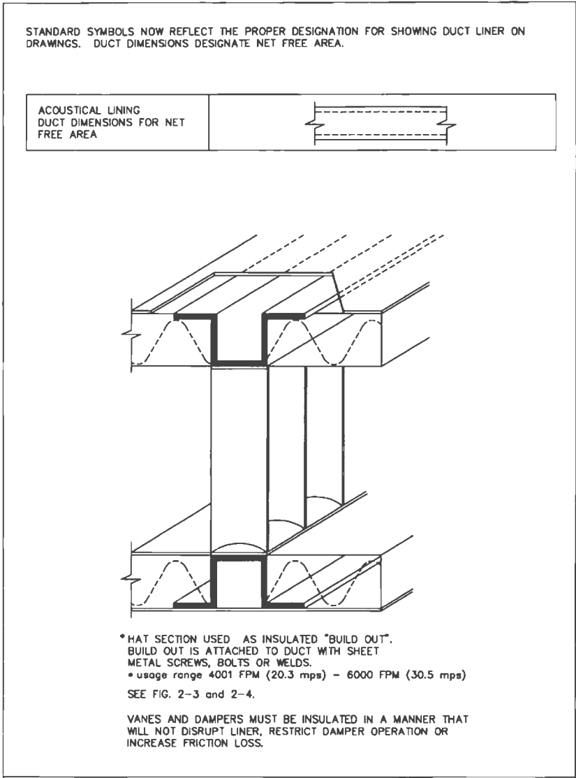
FIG. 2-21 OPTIONAL HAT SECTION
