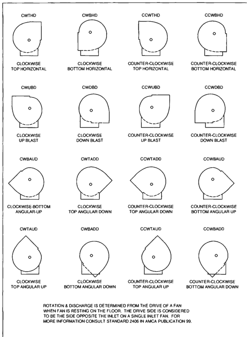
FAN ROTATION & DISCHARGE POSITIONS
