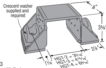
HGT-2 (HGT-3, HGT-4 similar)
