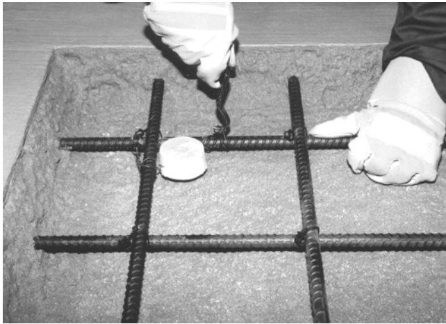
Fig. 7—Tying a Type 1A anode.
