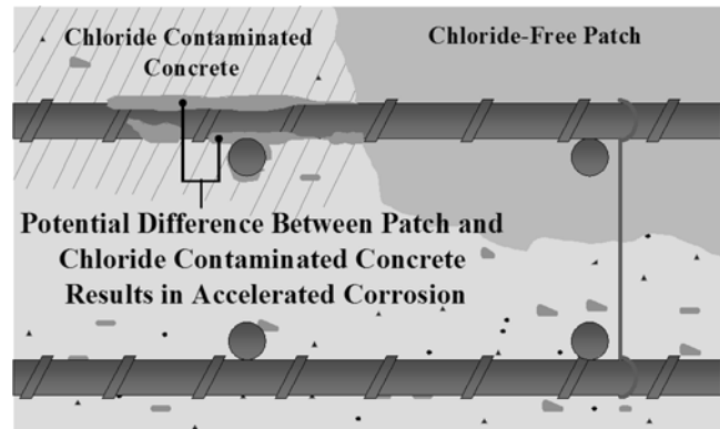
Fig. 1—“Ring-anode” corrosion.
