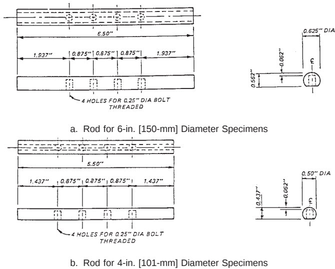
FIG. 6 Top Anvil Rods
