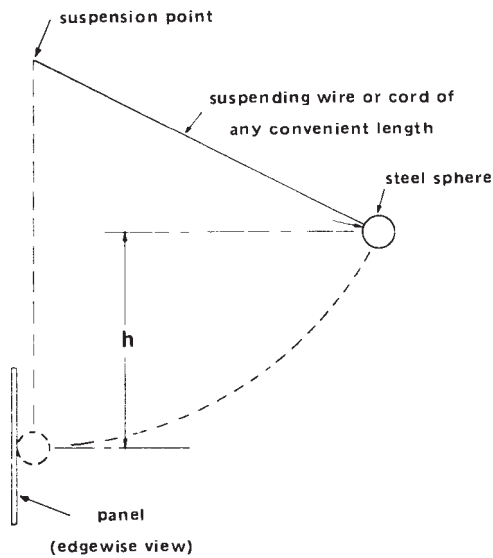
FIG. 7 Impact Test
