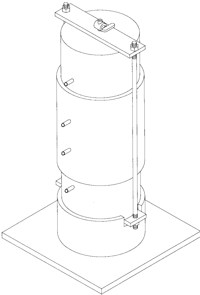
FIG. 1 Geotextile Permeameter
