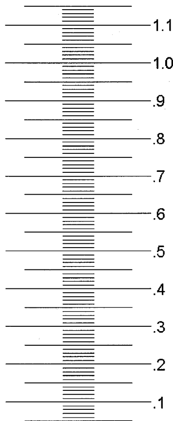
FIG. X1.1 Filar Scale
