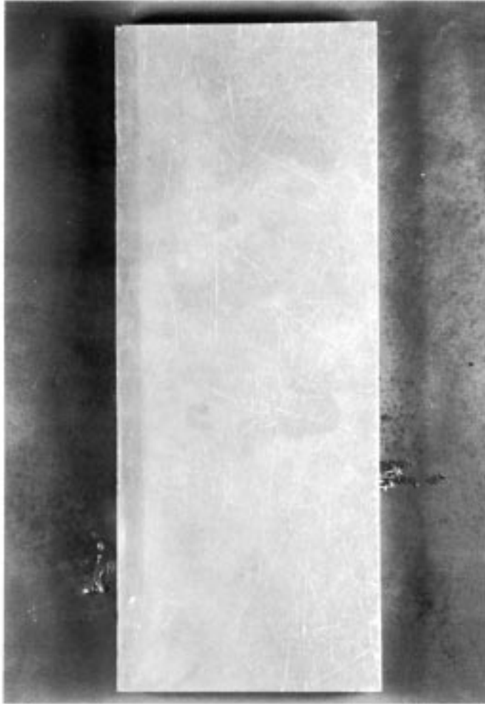
FIG. 16 Resin-Rich Edge
