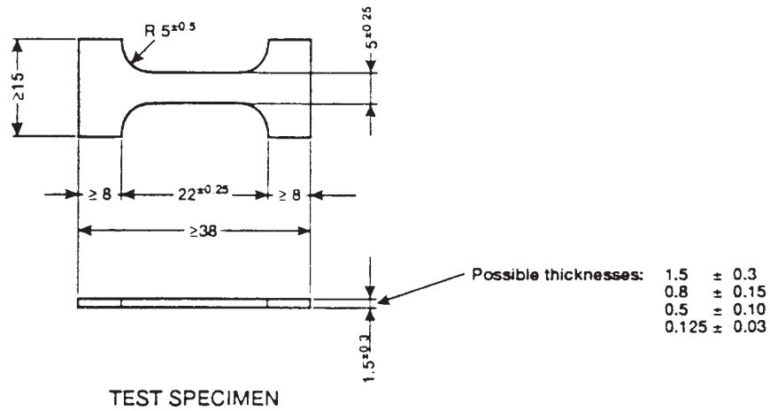
FIG. 1 Microtensile Die
