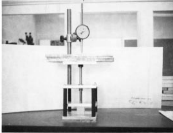
FIG. 2 Creep Test Apparatus
