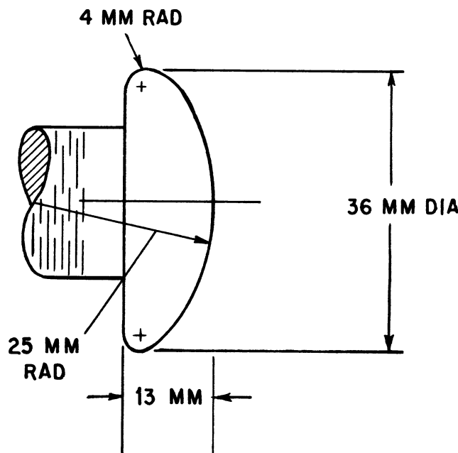
FIG. 1 VDE Electrode
