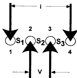
FIG. 1A Colinear Probe Array
