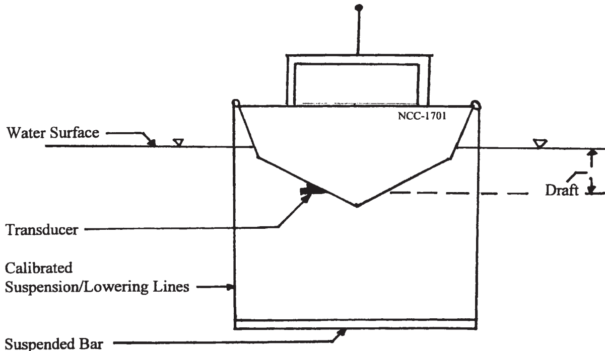
FIG. 1 Calibration Bar Apparatus
