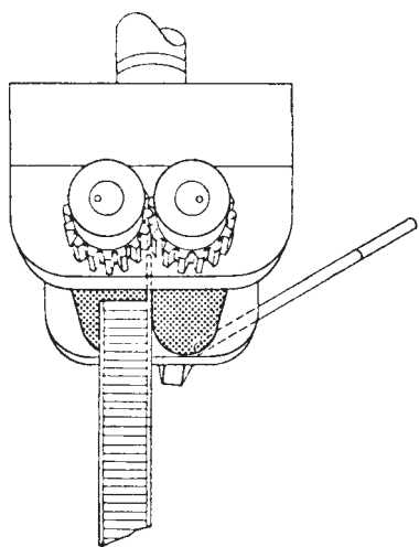
FIG. 2 Top Clamp
