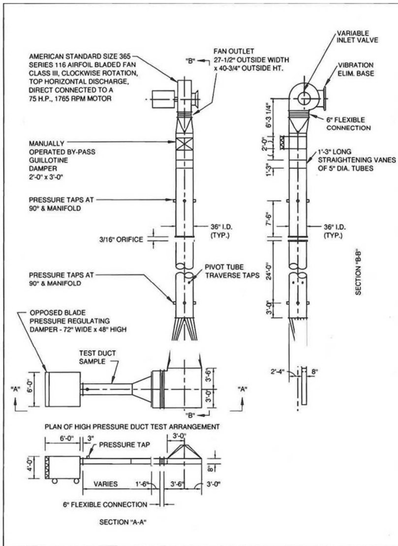
FIG. 7-4 TEST APPARATUS
