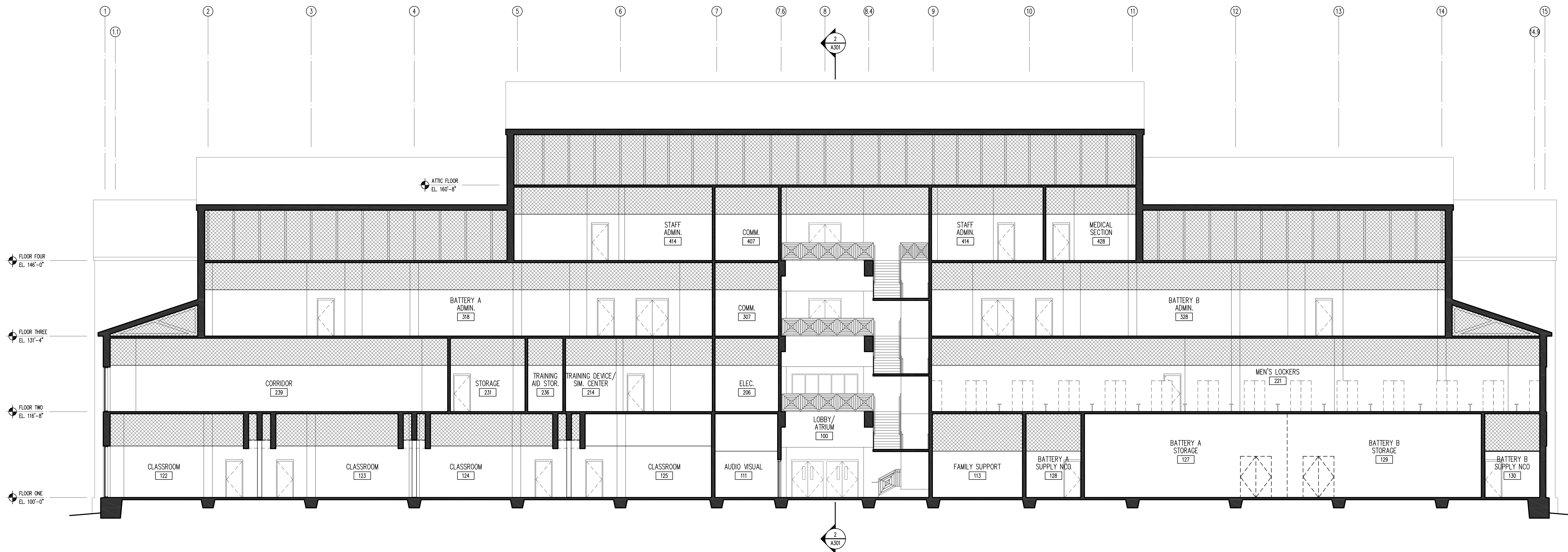
1 LONGITUDINAL BLDG. SECTION 1/8" = 1'-0"
