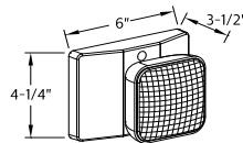
VLT1R dimensions
