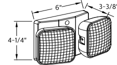
VLT2R dimensions
