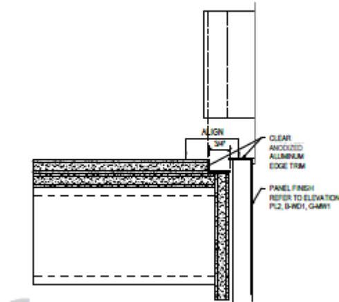
1 EDGE DETAIL
