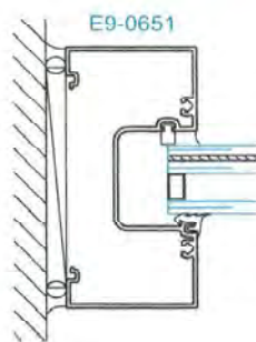
SECTION 4 JAMB
