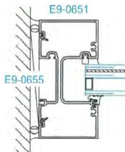
SECTION 4 JAMB
