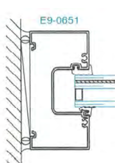
SECTION 4 JAMB
