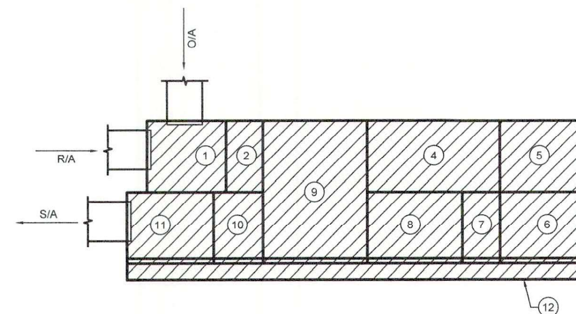
AHU-01 SCHEMATIC
