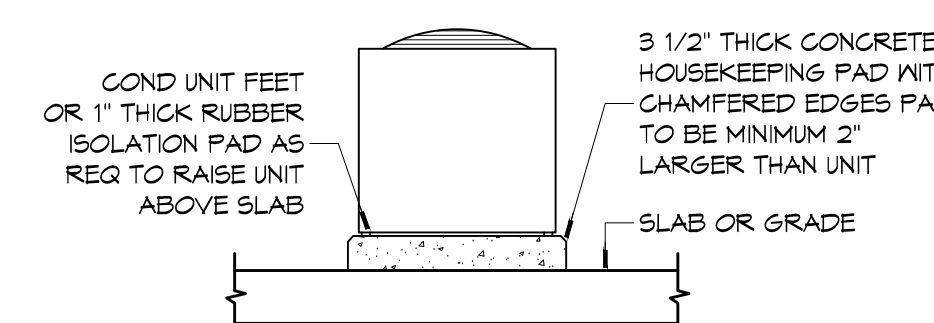
5 TYPICAL A/C CONDENSER DETAIL SCALE: N.T.S.
