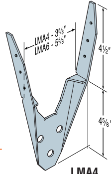
LMA4 (LMA6 similar)
